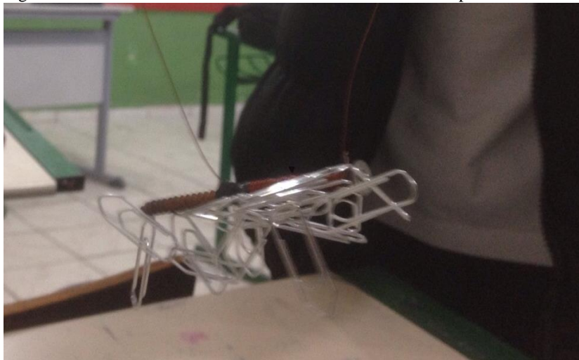
Figura 10 – Eletroímã em funcionamento durante a atividade experimental
