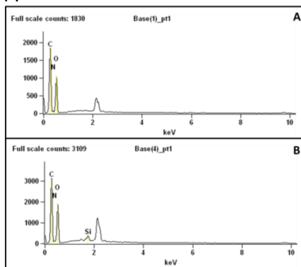
Figura 19: Análise de EDS das membranas de QTS, onde: A) QTS pura; B) QTS com NTS-F.
