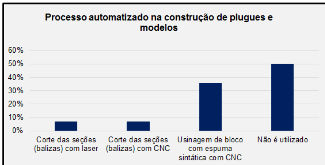
Figura E 2 – Processos automatizados para construção de plugues e modelos na região Sudeste.
