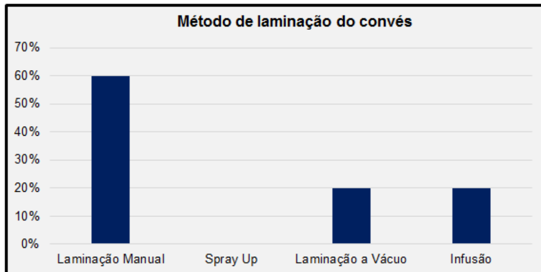
Figura F 4 – Método de laminação do convés na região Sudeste.
