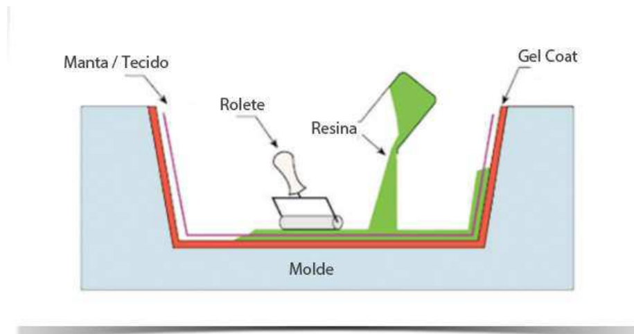
Figura 4 - Método de laminação Hand Lay Up
