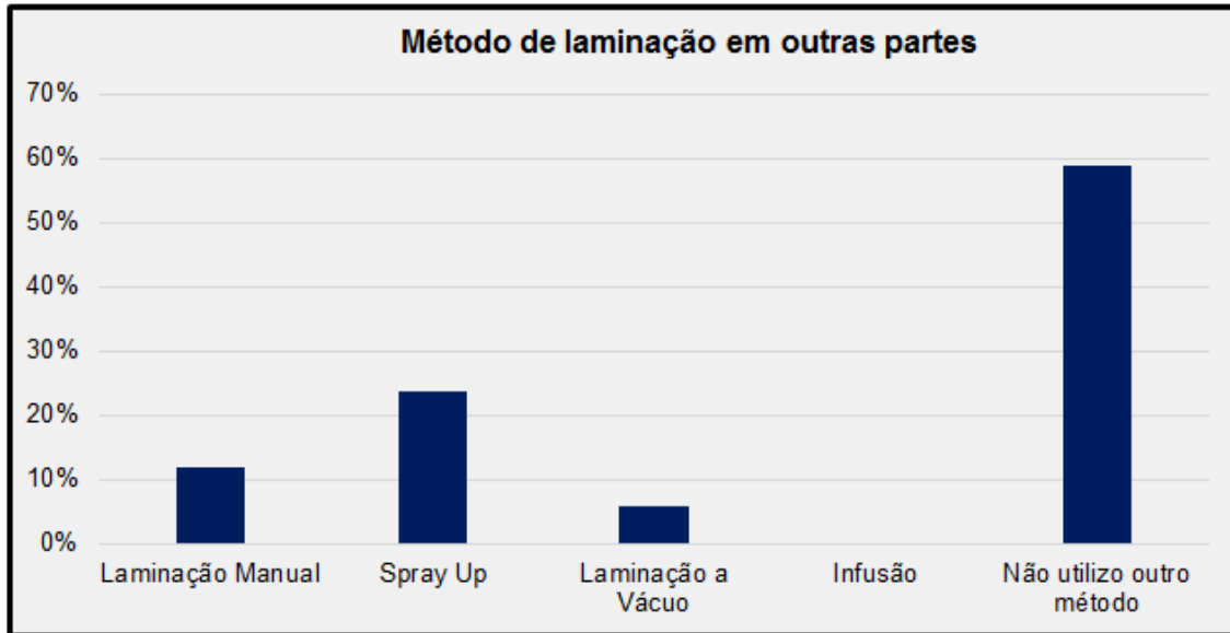
Figura F 5 – Método de laminação em outras partes da embarcação na região Sul.
