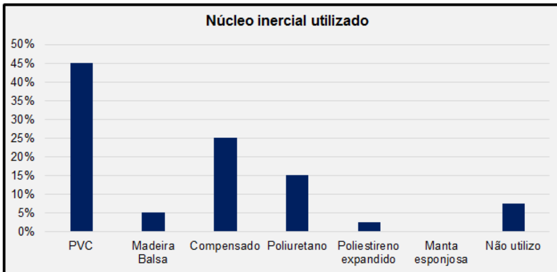
Figura J 1 – Núcleo inercial utilizado pelos estaleiros náuticos na região Sul.
