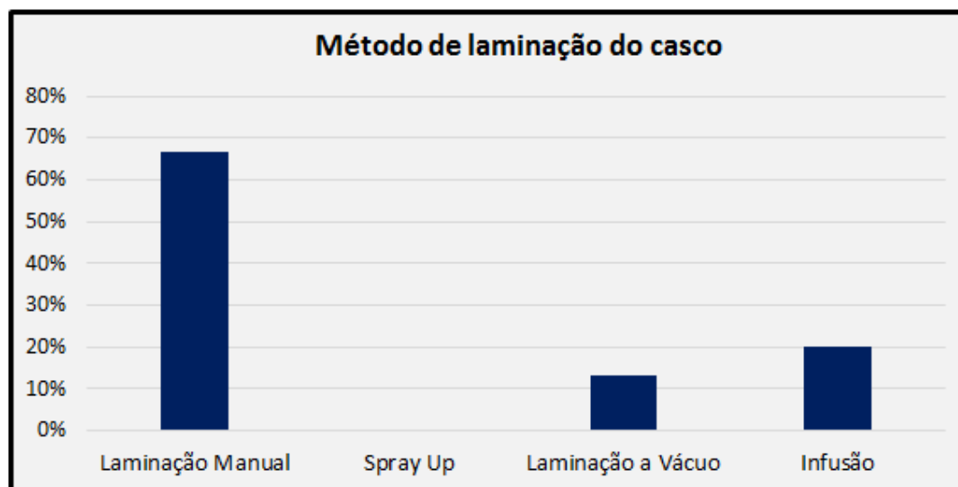
Figura F 2 – Método de laminação do casco na região Sudeste.
