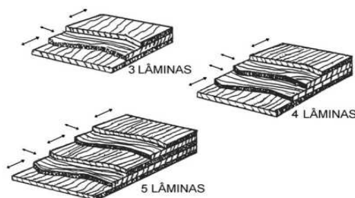
Figura 14 - Orientação das Laminas em Compensado Naval
