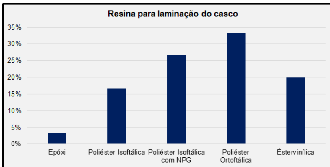
Figura 26 - Resina para laminação do casco
