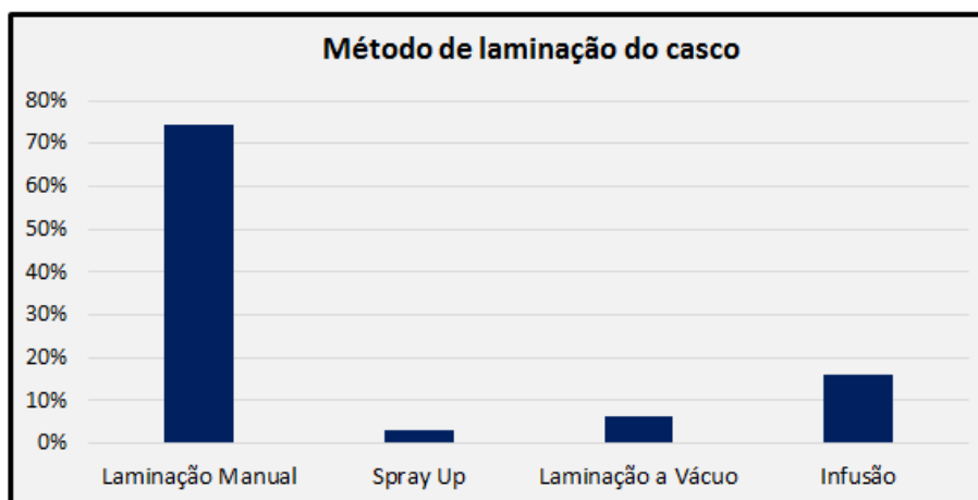
Figura 23 - Método de laminação do casco
