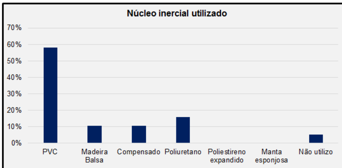
Figura J 2 – Núcleo inercial utilizado pelos estaleiros náuticos na região Sudeste.
