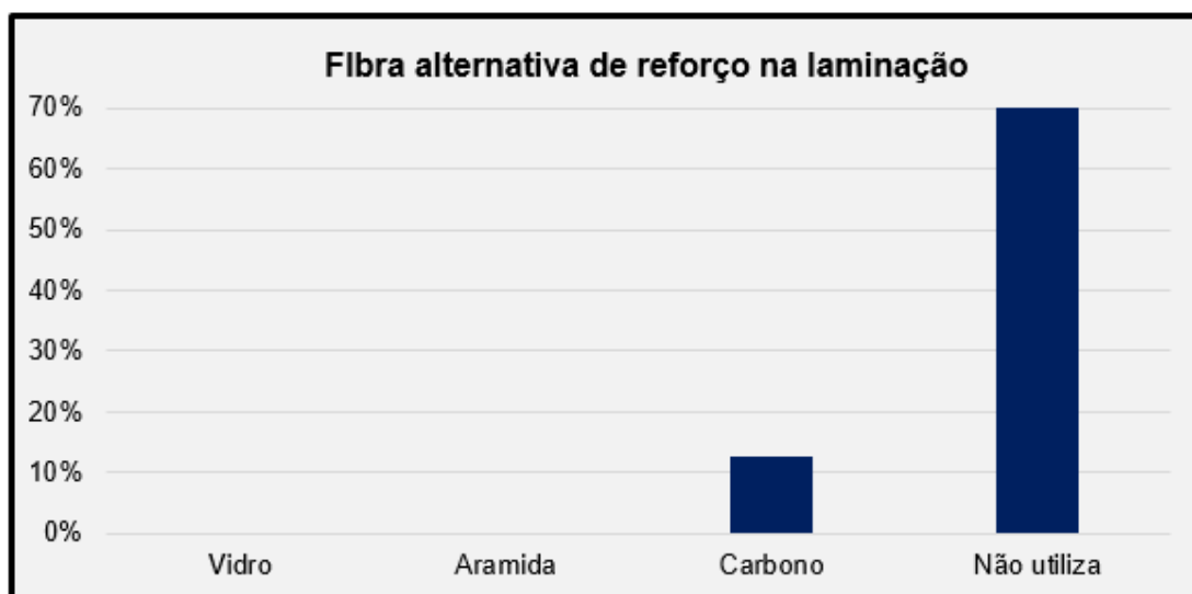
Figura I 3 – Fibras alternativas de reforço utilizadas nos estaleiros náuticos da região Sul.
