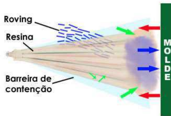
Figura 5 - Método de Laminação Spray Up
