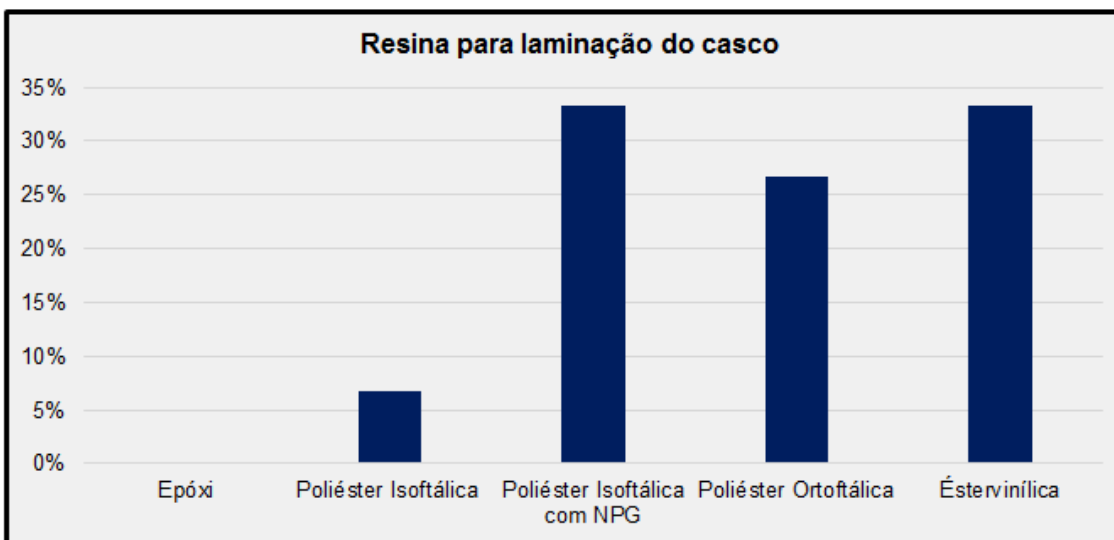
Figura G 2 – Resina utilizada para laminação do casco nos estaleiros da região Sudeste.
