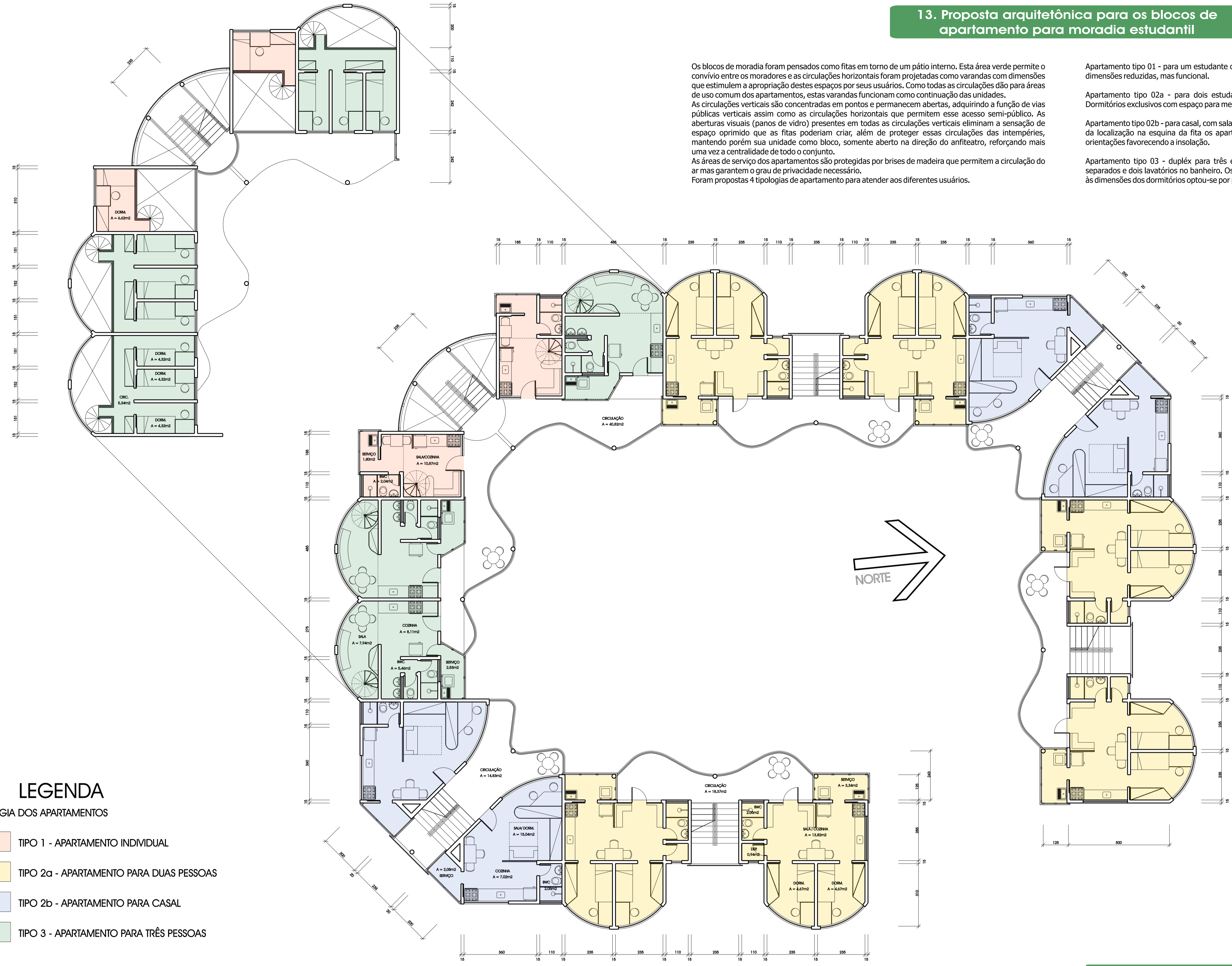
Planta Baixa - Pavimento tipo - Bloco Oeste
