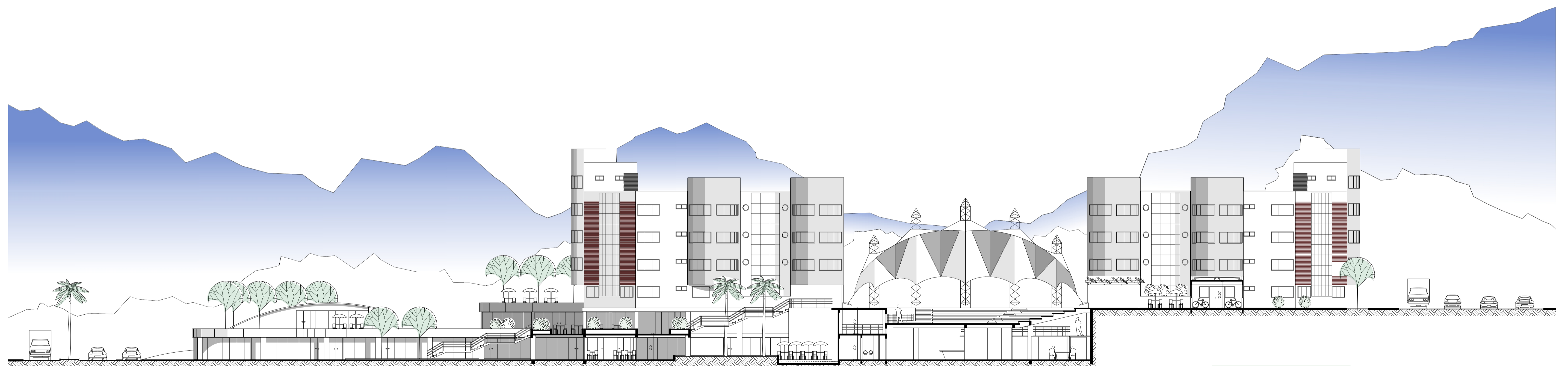
Corte B-B
