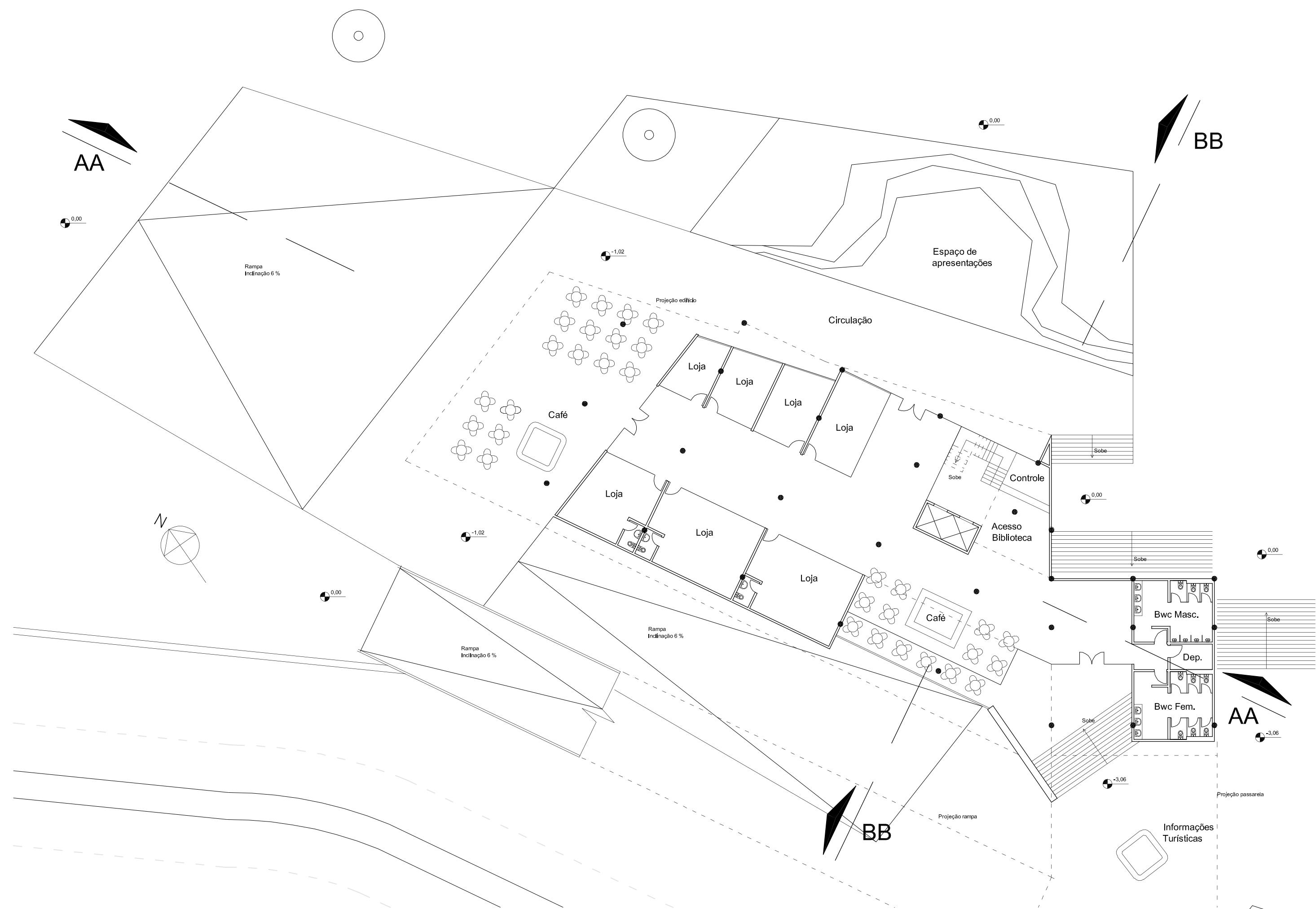
Planta Baixa Térreo Esc. 1/250
