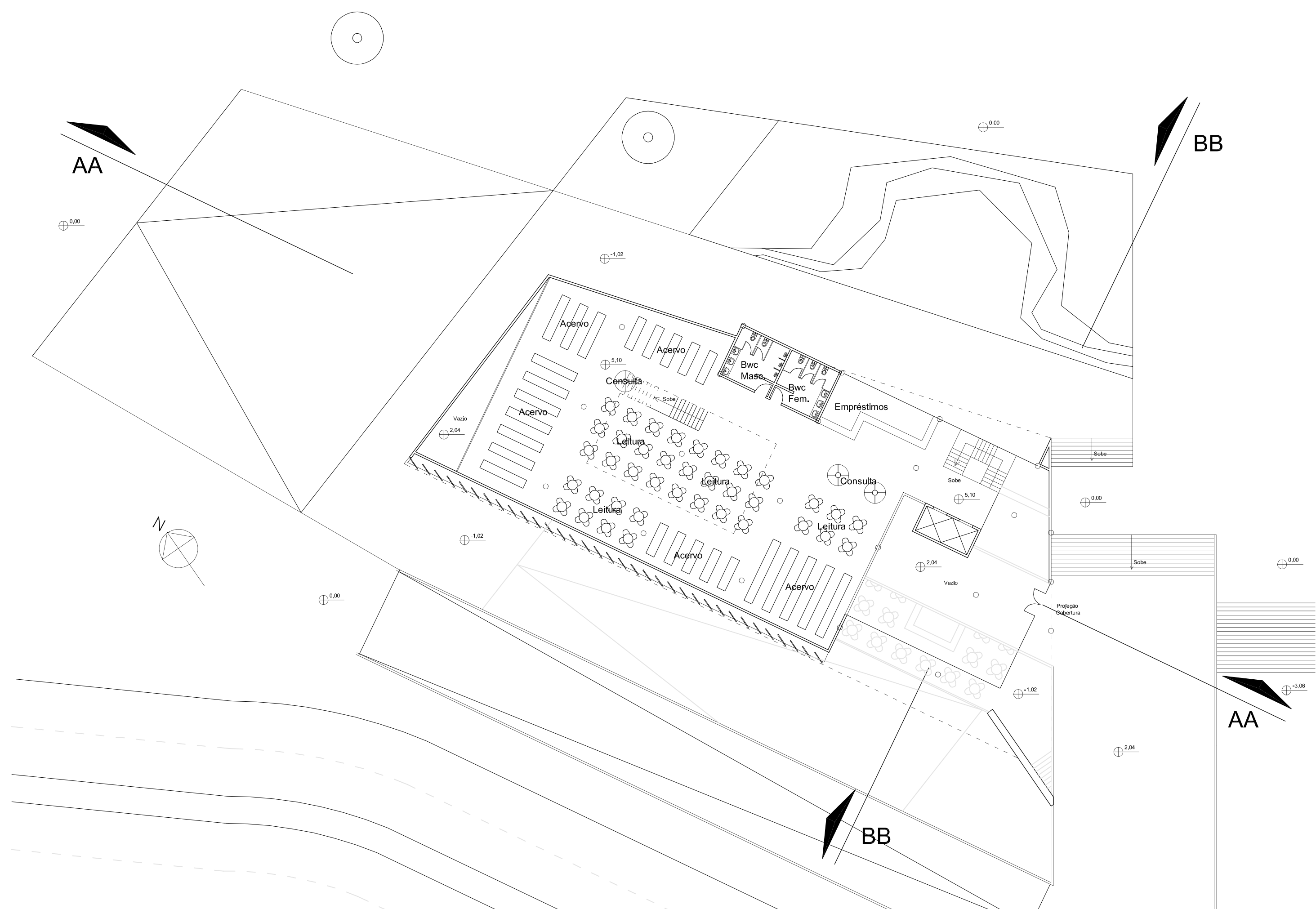
Planta Baixa 2o Pavimento Esc. 1/250
