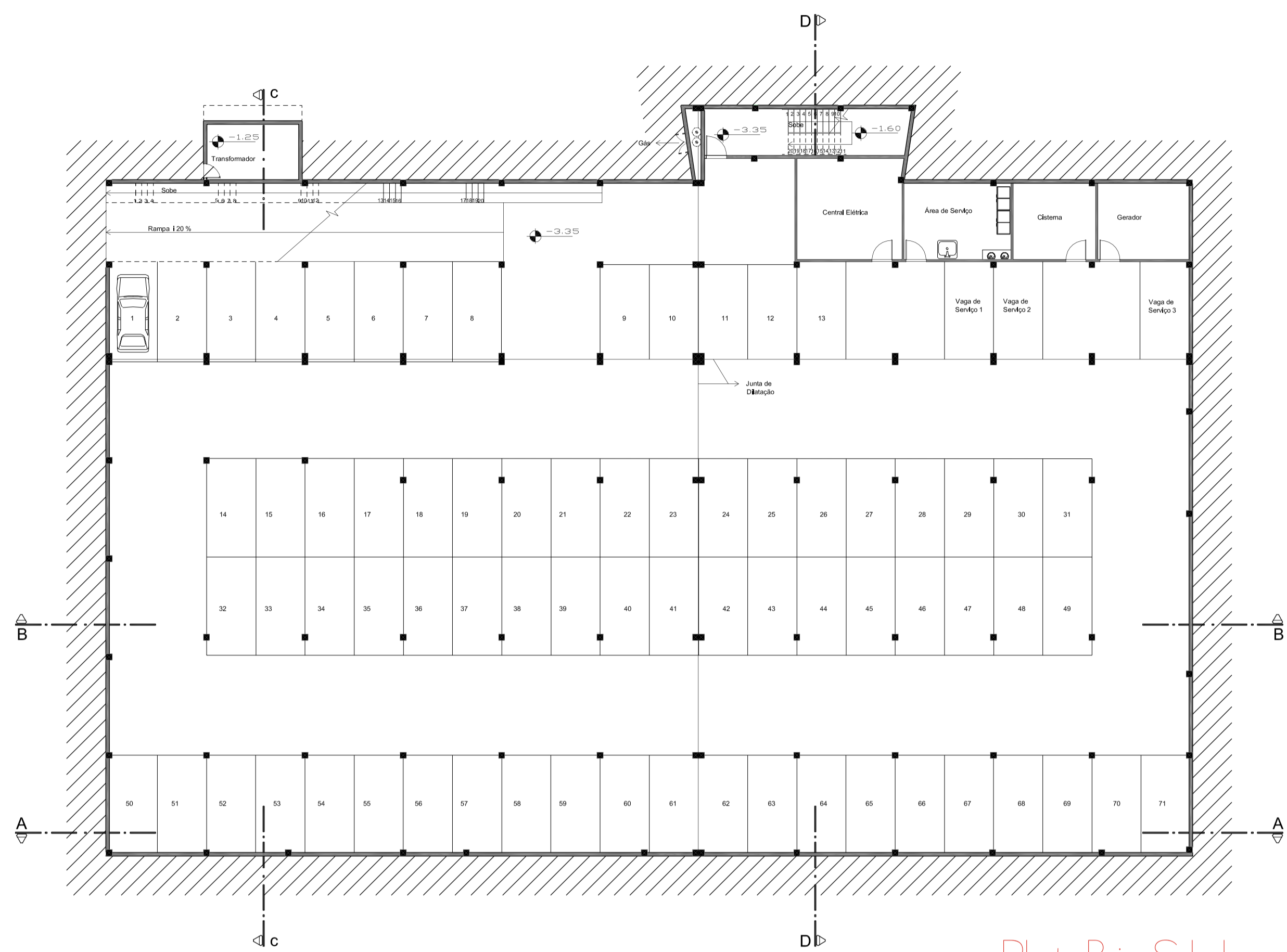
Planta Baixa Subsolo Esc: 1/200
