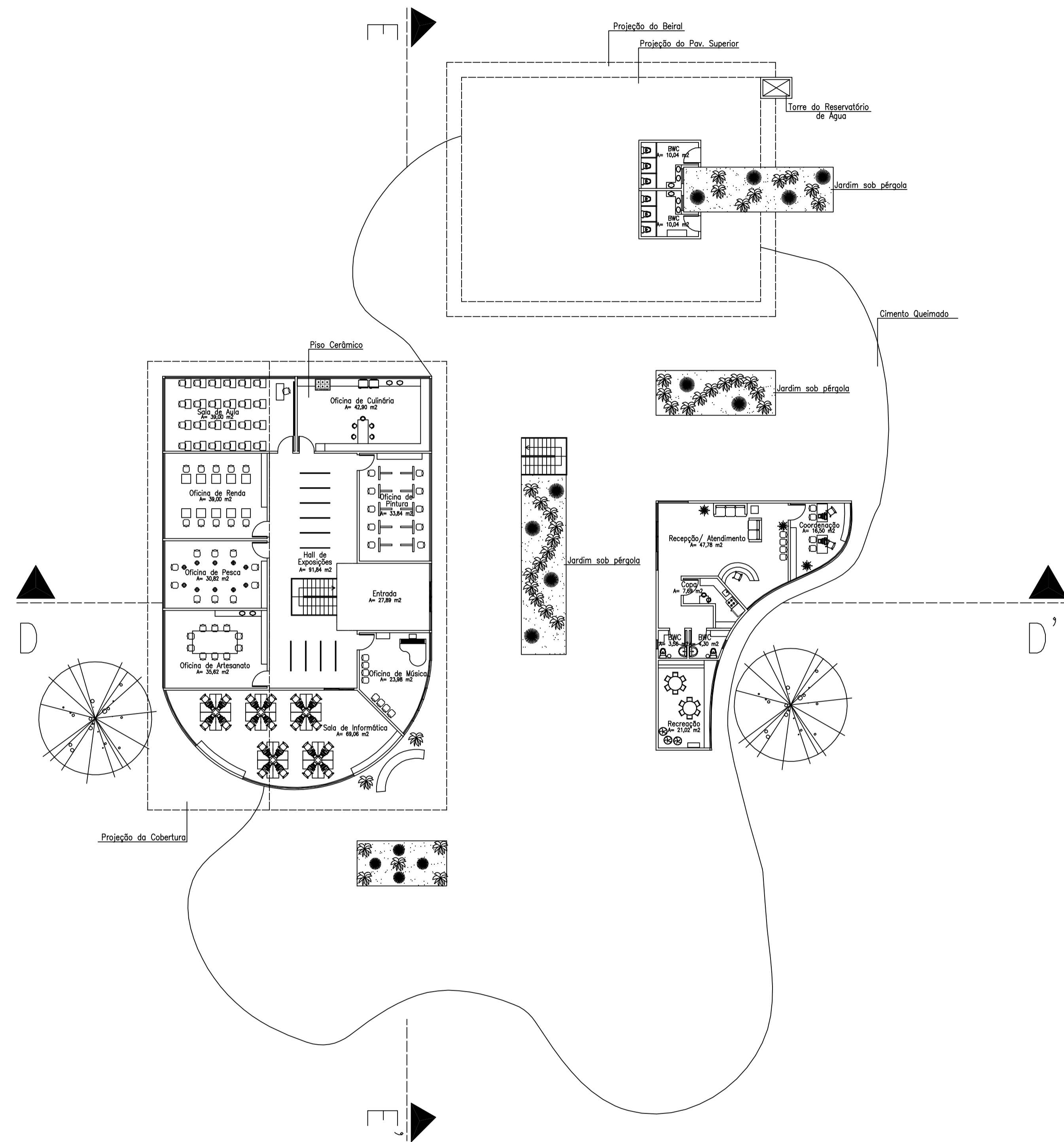
Planta - Baixa do Pav. Térreo Esc. 1/200
