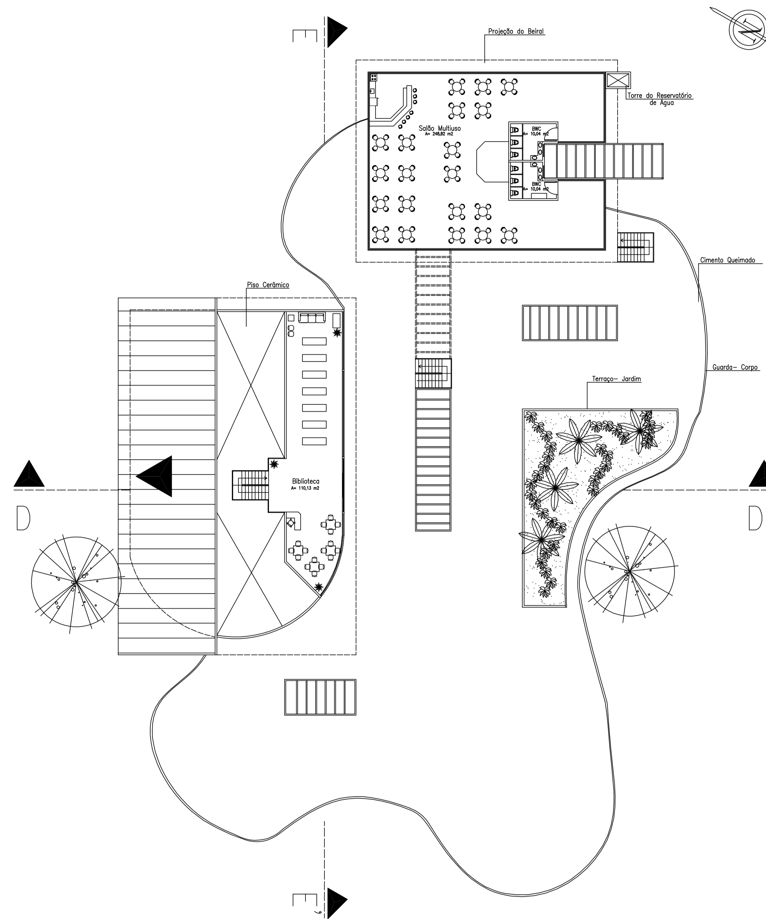
Planta - Baixa do Pav. Superior Esc. 1/200
