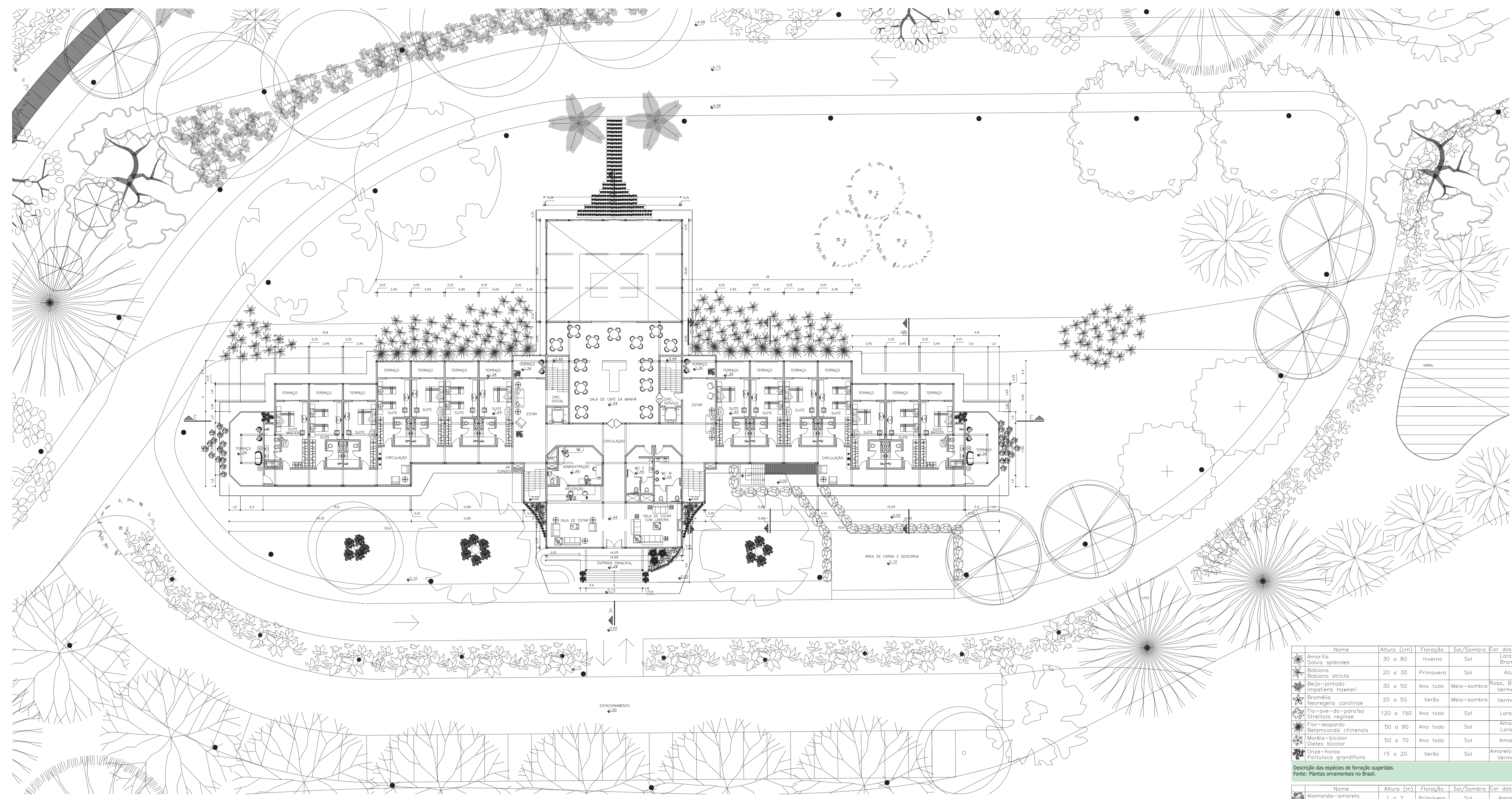
Planta Baixa Pavimento Térreo Esc. 1:200
