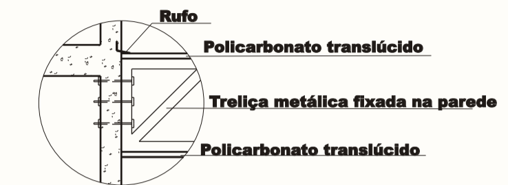
Detalhe 2 Escala gráfica 0cm 40cm 80cm 20cm 60cm 1m
