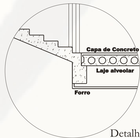
Detalhe 1 Escala gráfica 0cm 40cm 80cm 20cm 60cm 1m
