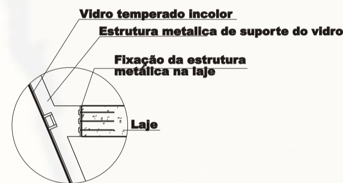
Detalhe 3 Escala gráfica 0cm 40cm 80cm 20cm 60cm 1m
