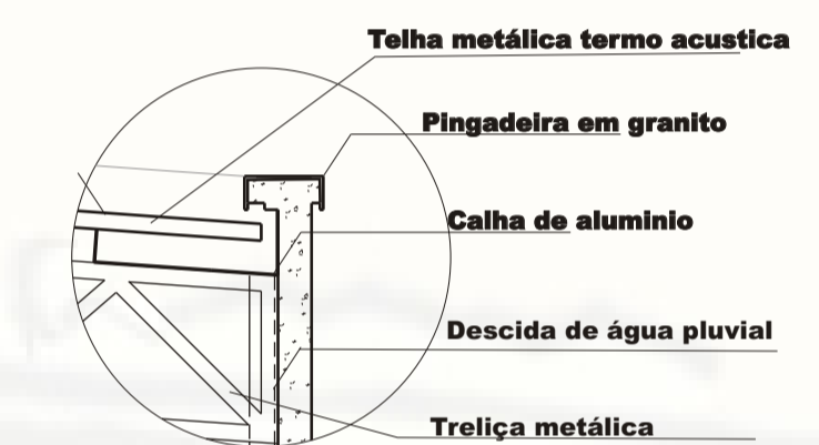
Detalhe 4 Escala gráfica 0cm 40cm 80cm 20cm 60cm 1m
