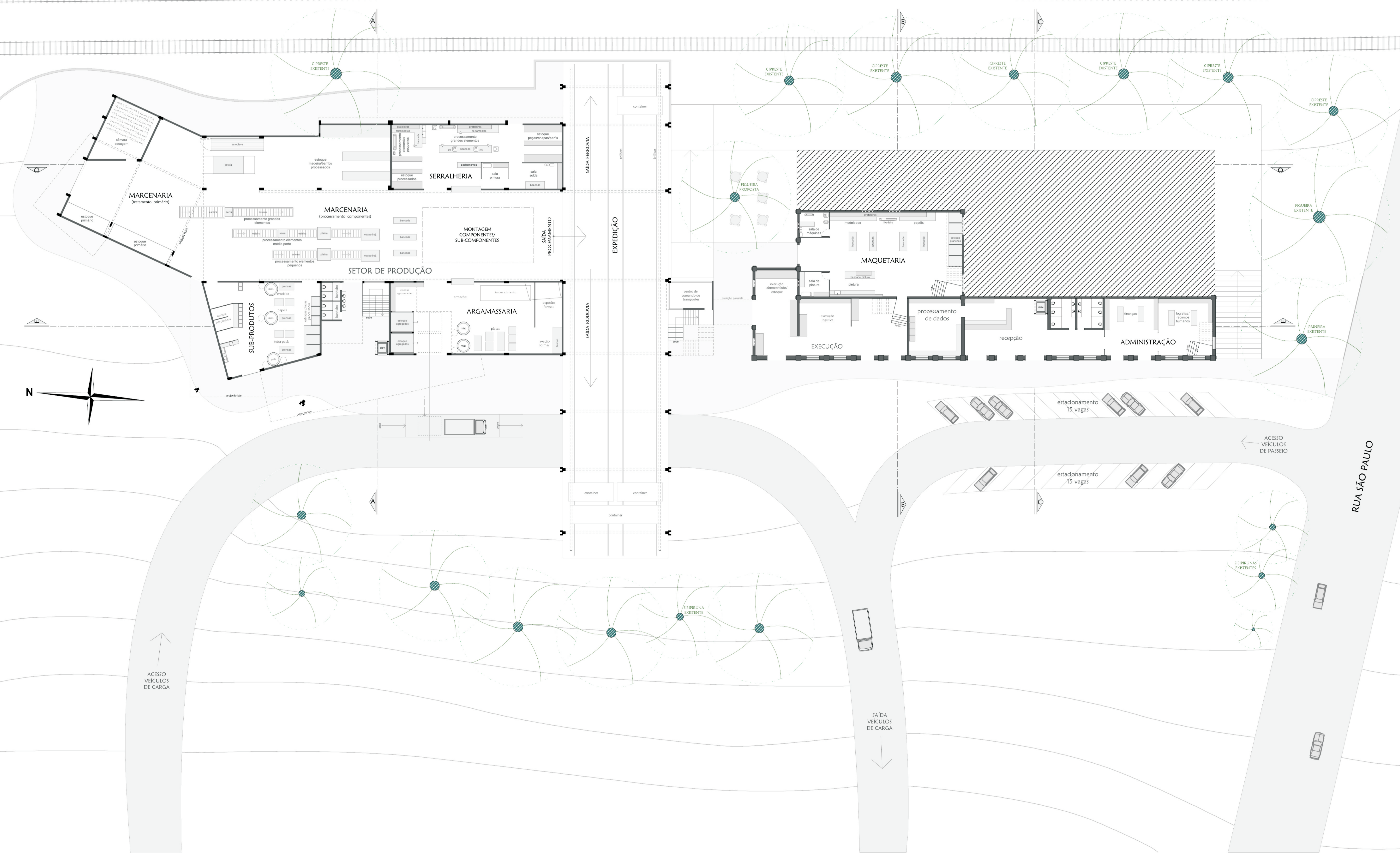
PLANTA PAVIMENTO TÉRREO SETOR DE PROCESSAMENTO E APROVEITAMENTO, E ESPAÇOS ADMINISTRATIVOS escala 1:250
