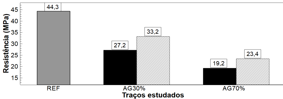
Figura 3 – Resultados do ensaio de compressão axial simples aos 91 dias. Na qual
