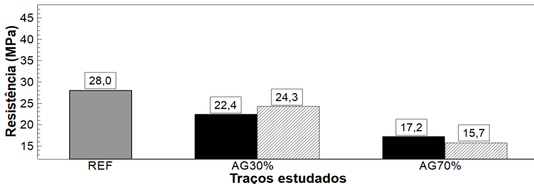
Figura 1 – Resultados do ensaio de compressão axial simples aos 7 dias. Na qual
