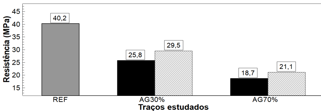
Figura 2 – Resultados do ensaio de compressão axial simples aos 28 dias. Na qual
