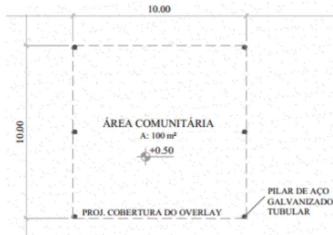
Figura 7: Planta baixa das áreas comunitárias. Fonte: Carbonari (2021).
