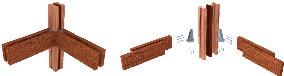
Figura 7. Interface pilar-2 vigas de canto. – Fonte: elaborado pelos autores
