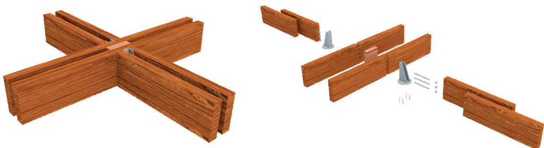
Figura 8. Interface viga-viga. – Fonte: elaborado pelos autores
