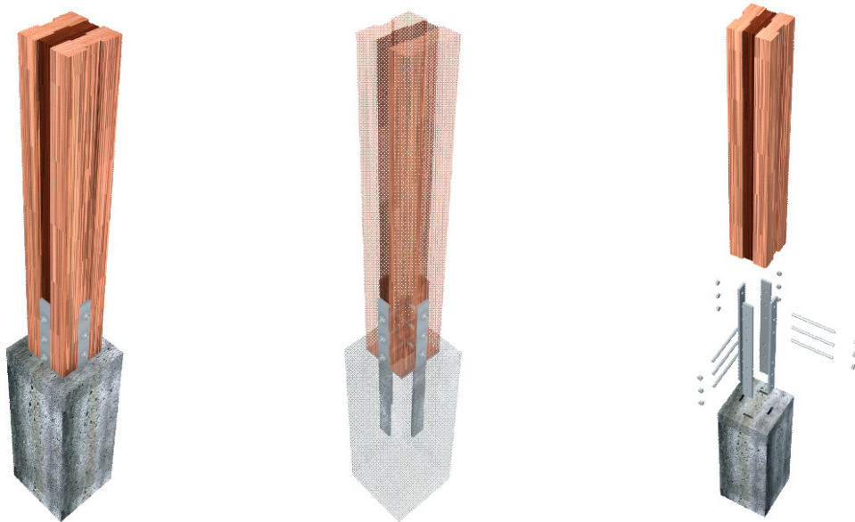
Figura 4. Interface pilar-fundação. – Fonte: elaborado pelos autores
