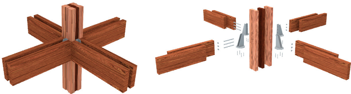
Figura 5. Interface pilar-4 vigas. – Fonte: elaborado pelos autores
