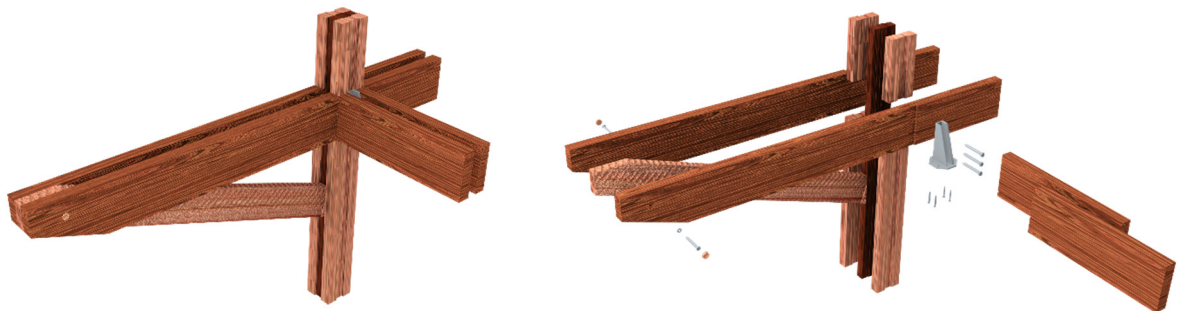
Figura 6. Interface pilar-2 vigas com mão francesa. – Fonte: elaborado pelos autores
