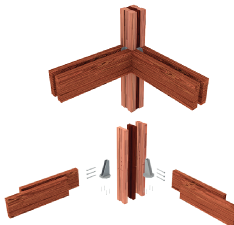
Figura 07 – Interface pilar-2 vigas duplas de canto
