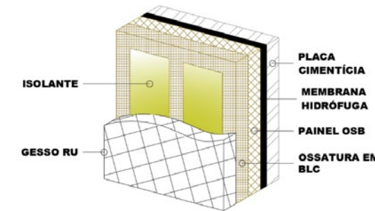
Figura 8: Vedação com placa cimentícia e gesso RU. Fonte: elaborado pelos autores.
