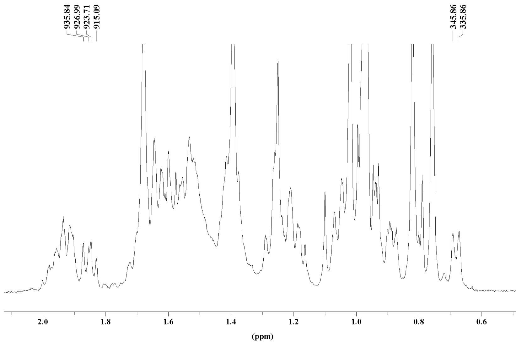
Figura 18. Detalhes ampliados da região de campo alto do espectro de RMN de próton de ZI2 em \text{CDCl}_3 (300 MHz).
