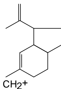
Figura 10. Estrutura do fragmento correspondente ao pico-base em m/z = 203 no espectro de massas de triterpenos, segundo OGUNKOYA (1981).
